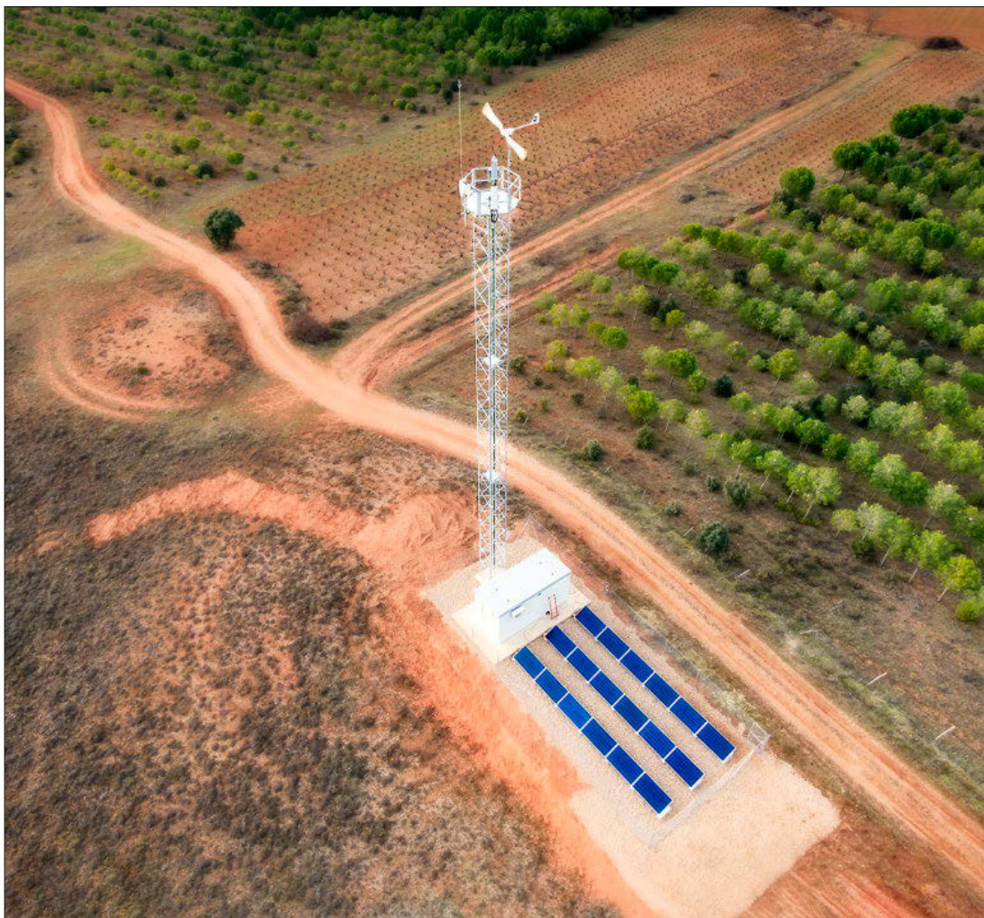
Antena para dar cobertura 5G y banda ancha en Matanza de Soria junto a sus instalaciones auxiliares. HDS
